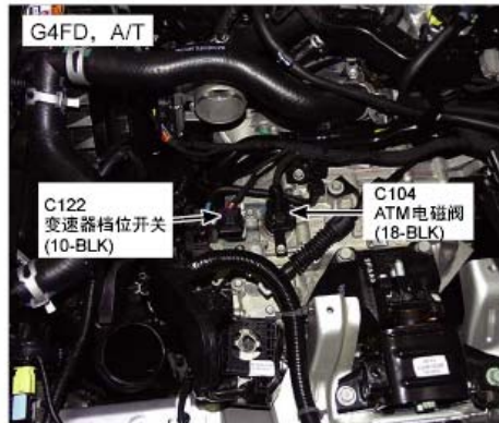
45. 变速器顶部
