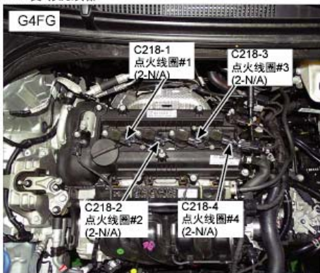
47. 发动机顶部
