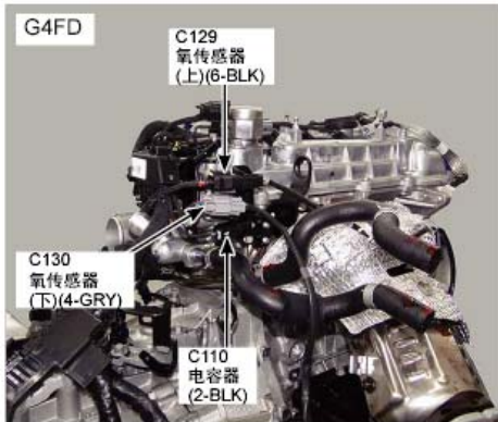
43. 发动机后右
